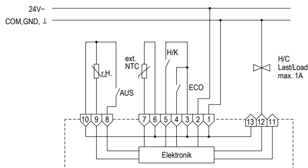
KTRRB-052.24x Anschluss im 2-Rohr-Leitungssystem
