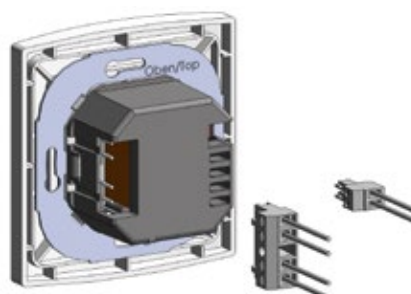
steckbare Schraubklemmen
