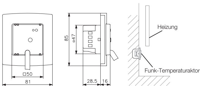
Aktor 50 x 50 mit Alre-Rahmen
