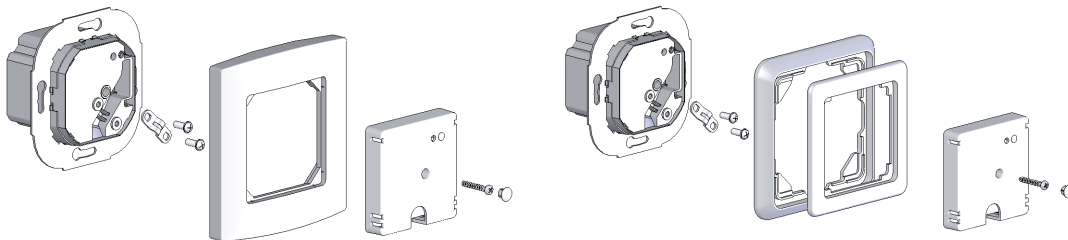
Aktor 50 x 50 mit Alre-Rahmen
